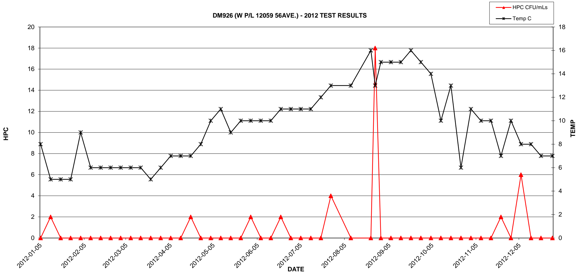
DM926 (W P/L 12059 56AVE.) - 2012 TEST RESULTS
